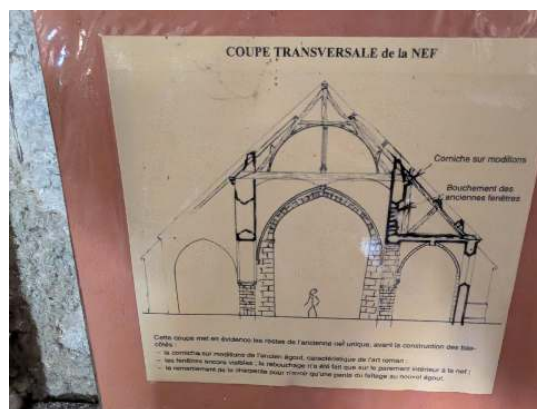
Coupe transversale de la nef mettant en évidence les restes de l'ancienne nef unique romane dans les combles (corniche sur modillons et fenêtres obturées).
